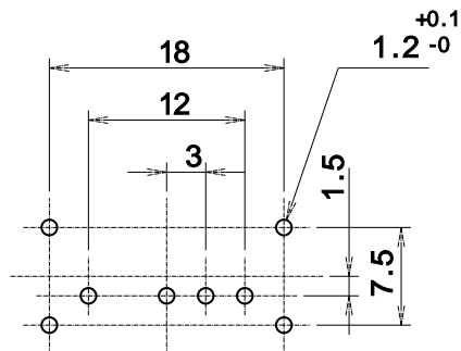
基板取付穴参考寸法 (S=2/1) (スイッチ取付面より) (一般公差 \pm 0.1 )
