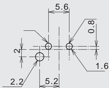
取付穴参考寸法 (S= 2/1) Mounting Hole
