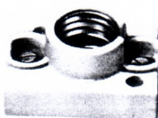
Plug-Fuse Cut-out, WK-501 1P 250V/30A WK-502 2P 250V/30A WK-503 3P 250V/30A
